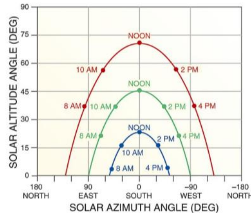
SUN PATHS FOR 45°N LATITUDE
