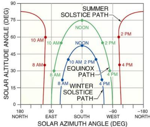
SUN PATHS FOR 15°N LATITUDE
