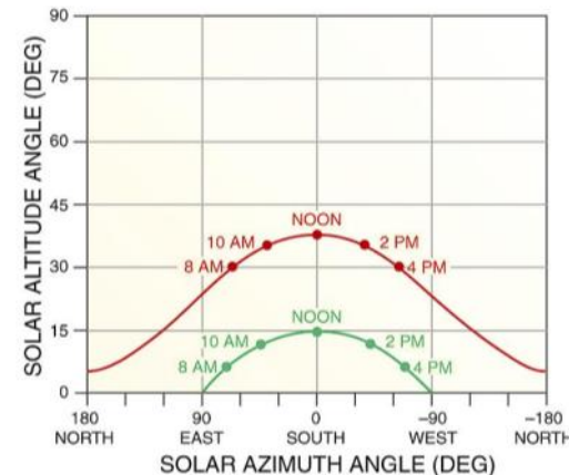
SUN PATHS FOR 75°N LATITUDE
